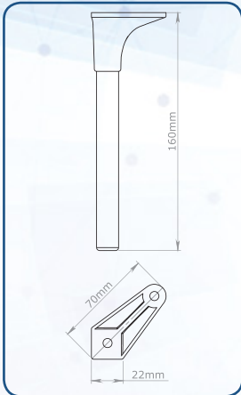
LIMON (15x160) mm 121119201110562 Krom - Antik Bronz
