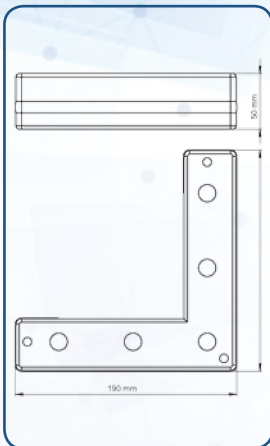
PELESENK (190x190x50) mm 111115612121362 Ağaç
