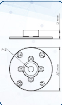
ARMUT ÜST BAĞLANTI 112651381348363 Siyah
