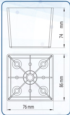
İNCİR (86x86x80) mm 111118412122562 Ağaç
