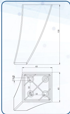
MEŞE (65x65x130) mm 111127201121462 Ağaç
