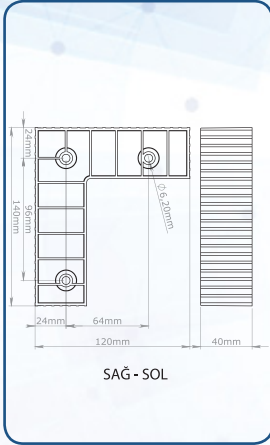
GÖKNAR (120x140x40) mm 111105101155262 Ağaç
