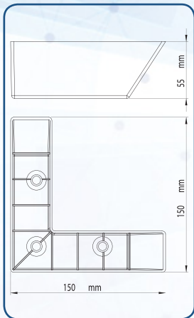
SEDİR (150x150x55) mm 111116412121463 Ağaç
