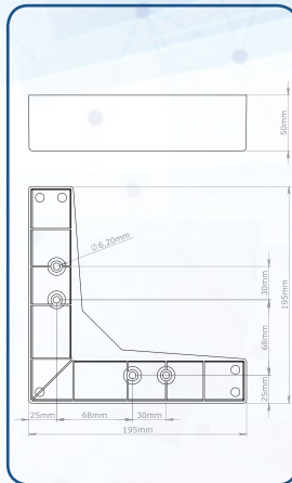
GÖKNAR (195x195x50) mm 111105812121462 Ağaç
